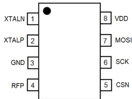
Figure2.2 YH350B SOP8 package
